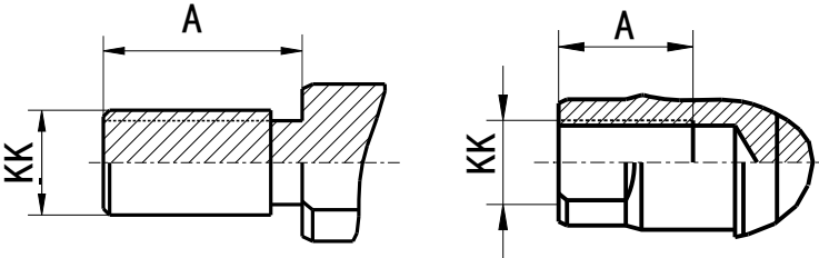
活塞杆端螺纹结构
