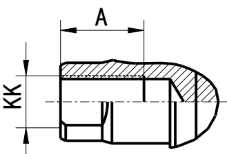
活塞杆端螺纹结构
