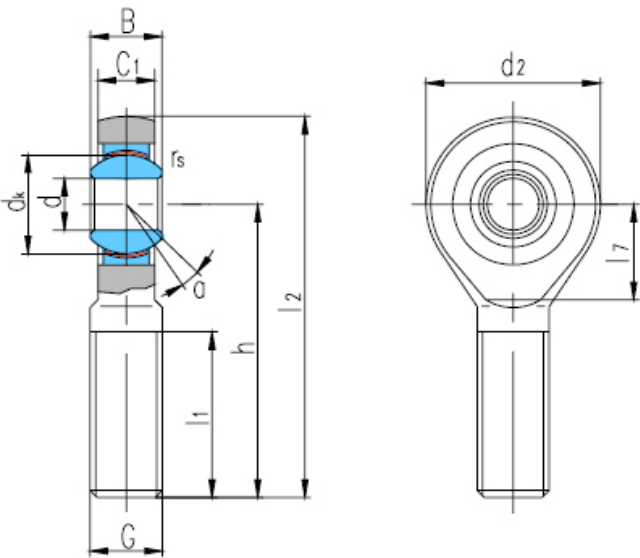
SA杆端轴承
