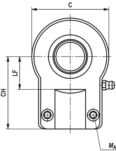
GIHO-K***-D0吊环头
