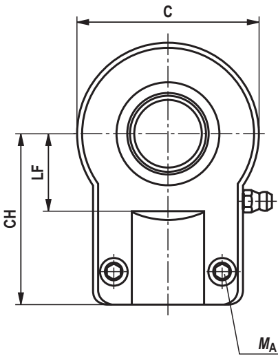
GIHO-K***-DO吊环头
